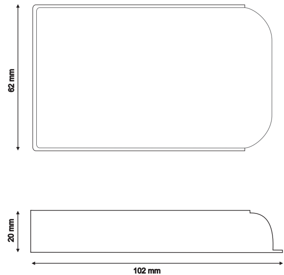
Halterung
